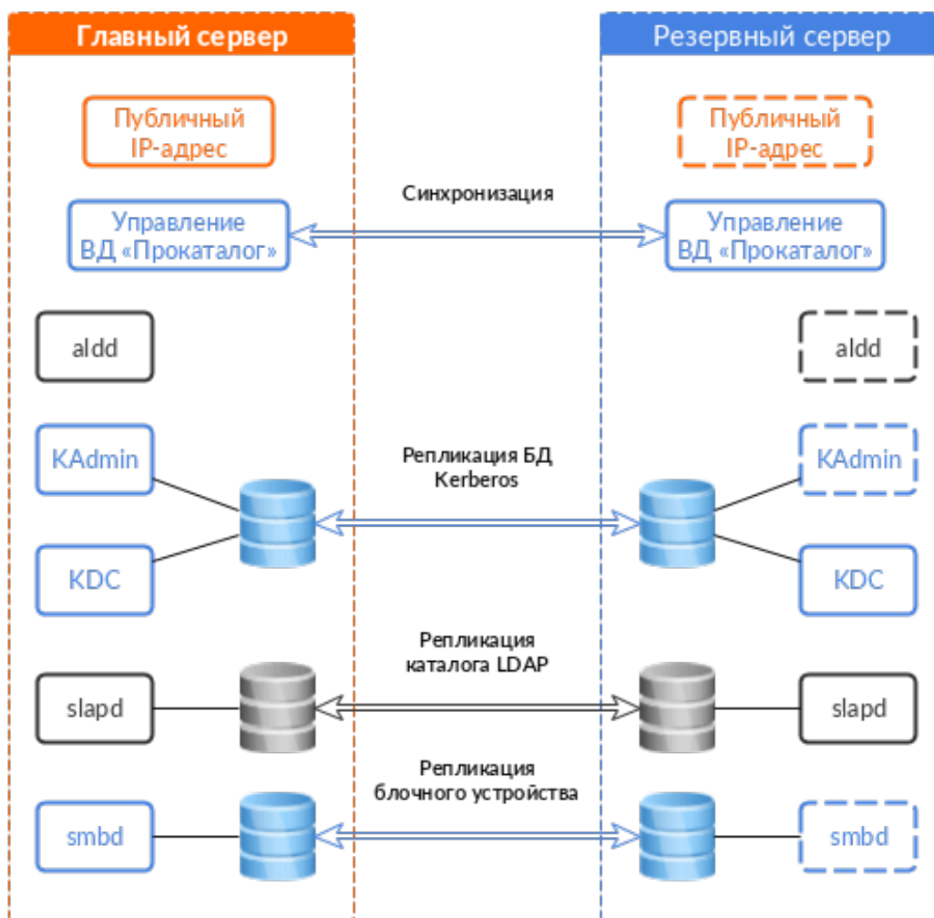
Рис. 3.1: Структурная схема ВД «Прокаталог»
